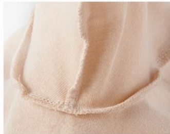
一般的な肌着の縫製(肌側)
